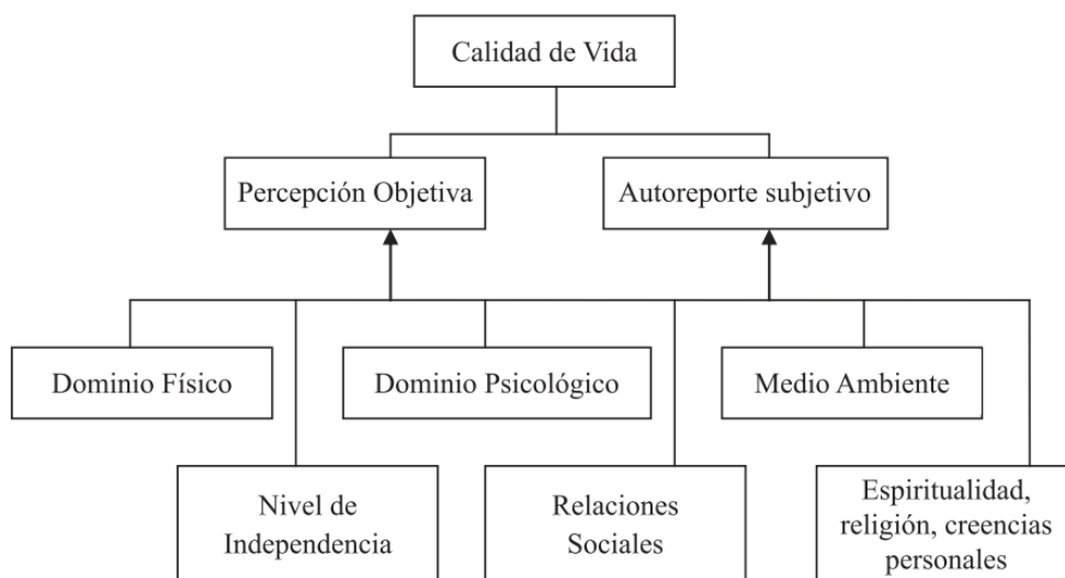
Figura 2 Diagrama del modelo conceptual de la Organización Mundial de la Salud.
