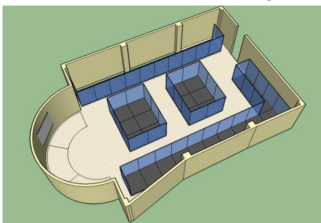
Figura 22. Modelo 3D, del espacio de exposición de los bienes muebles culturales de la Virgen.
