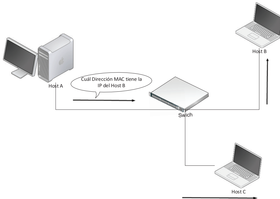
Figura 1: El Host A envía un broadcast ARP al host B.
