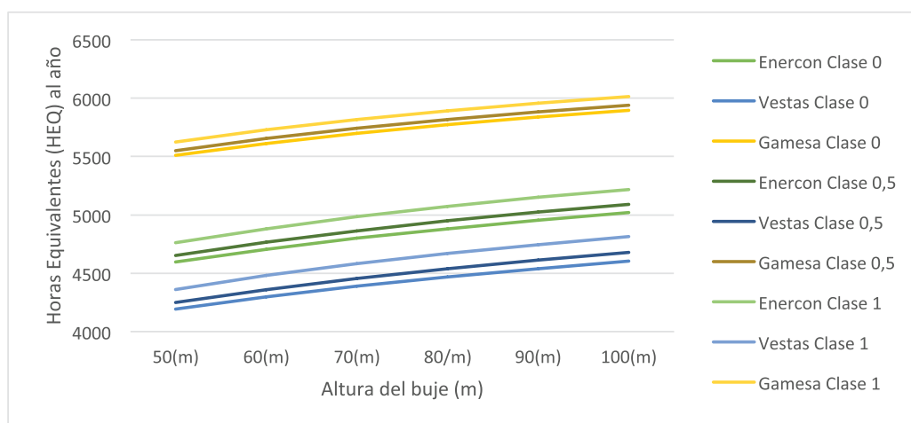
Figura 4. Comparación de las horas equivalentes producidas por tres aerogeneradores a diferentes alturas y clases de terreno
