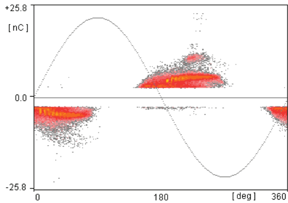
Figura 2. Descarga de tipo barra-barra
