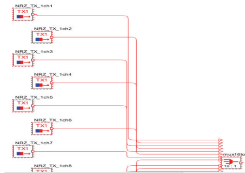
Figura 2. Ssistema Transmisor y uso de multiplexador
