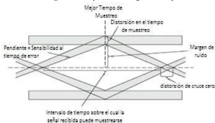
Figura 5. Esquema del diagrama de ojo
