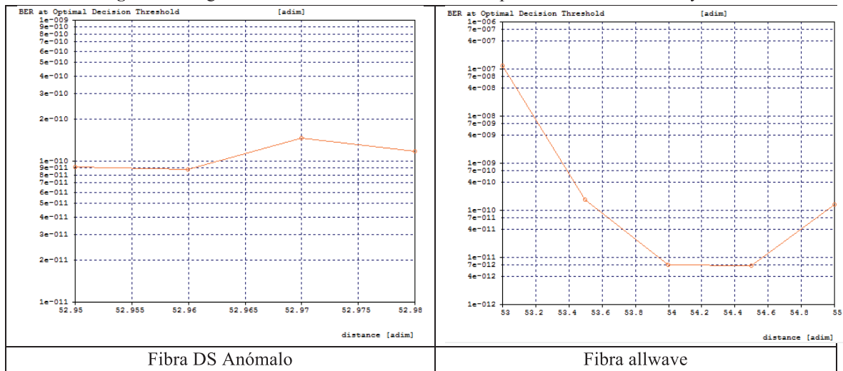
Figura 7. Diagramas de correlación BER-Distancia para fibras DS Anómalo y Allwave
