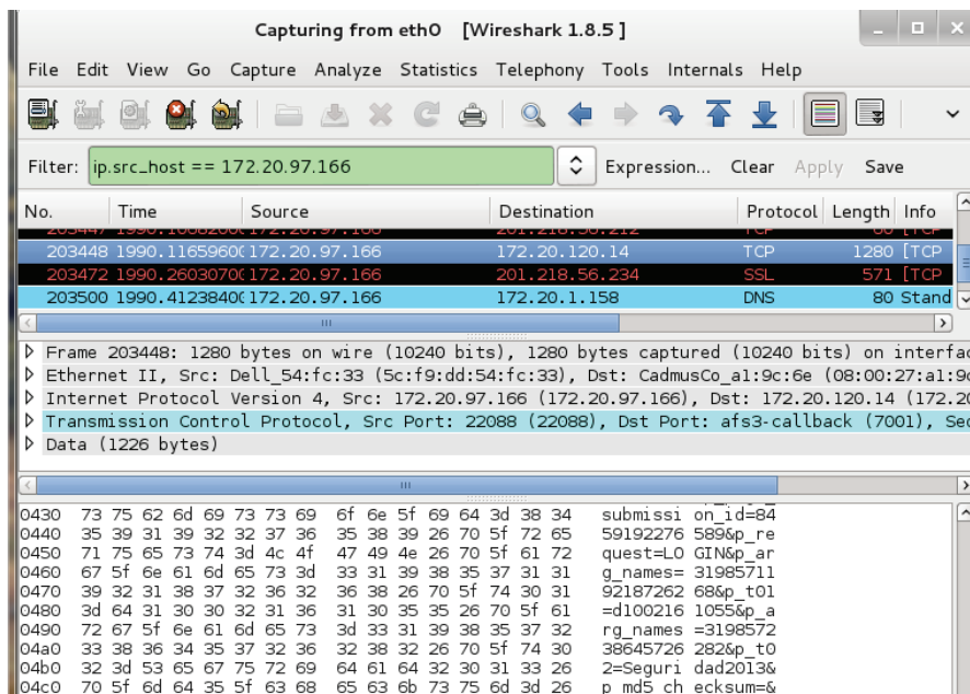
Figura 10: Resultado de la captura de claves cuando se usó HTTP.
