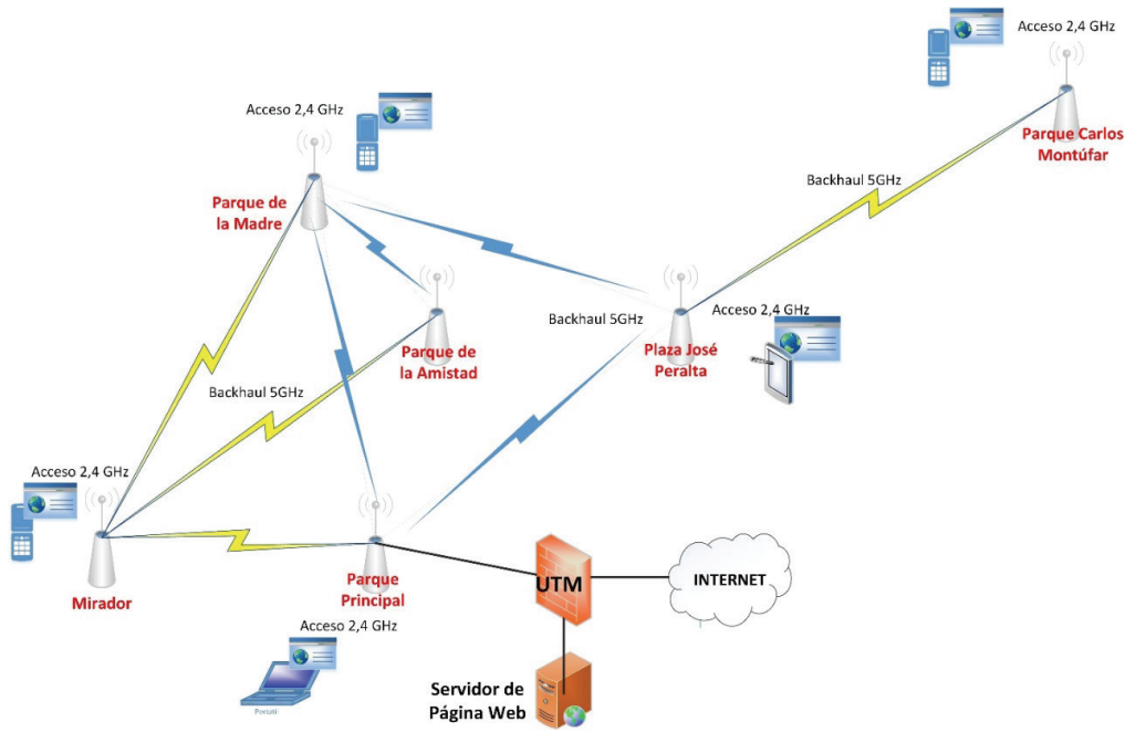
Fig. 1: Diagrama de la solución propuesta
