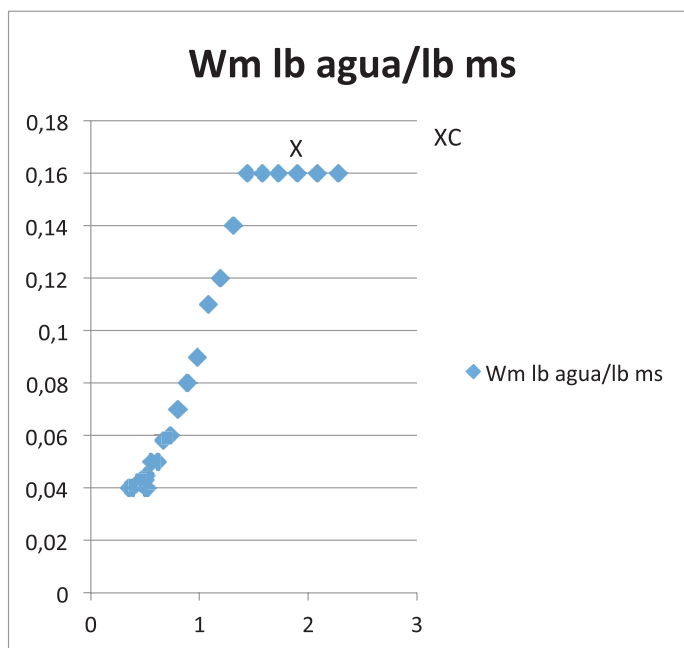
Figura 9: Wm lb agua / lb masa seca
