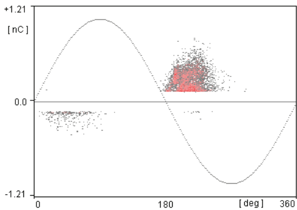
Figura 3. Descarga del tipo corona
