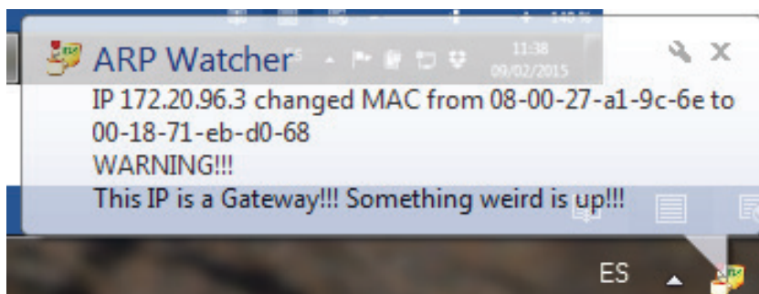
Figura 11: Detección del ataque ARP Spoofing por parte de la herramienta Decaffeinatid.
