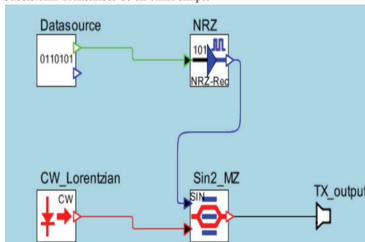
Figura 1. Subsistema Transmisor de un canal simple
