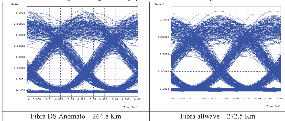
Figura 8. Diagrama del ojo para las fibras DS Anómalo y Allwave
