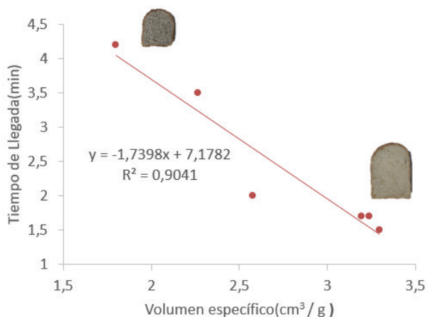
Figura 5. Correlación entre volumen específico y tiempo de llegada
