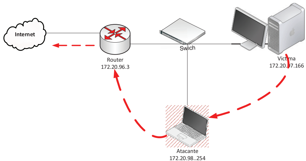
Figura 6: Topología después del ataque ARP Spoofing.
