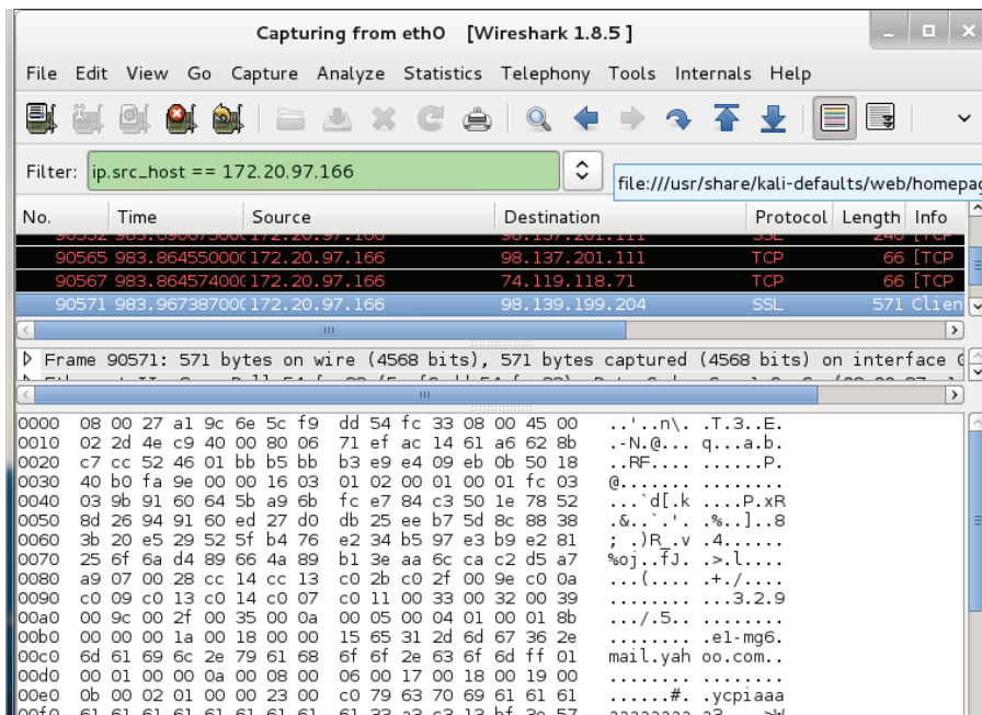
Figura 9: Resultado de la captura de claves cuando se usó HTTPS.
