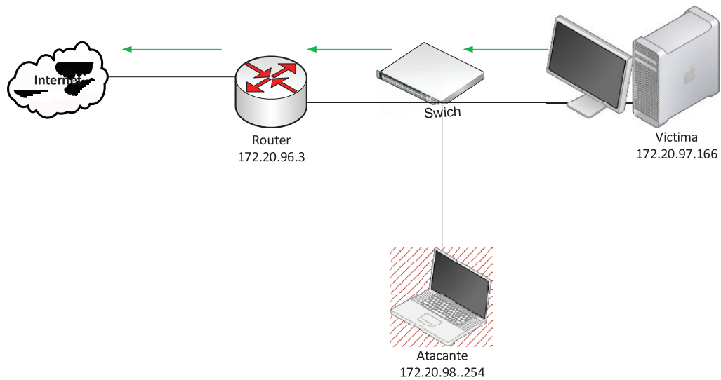
Figura 5: Topología antes del ataque ARP Spoofing.
