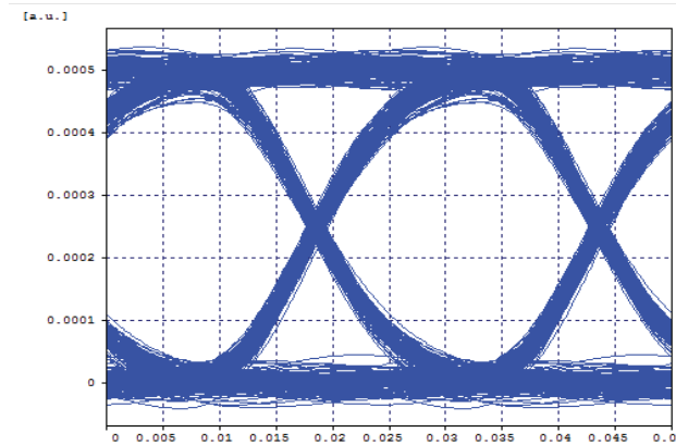
Figura 6. Diagrama de ojo en el backtoback
