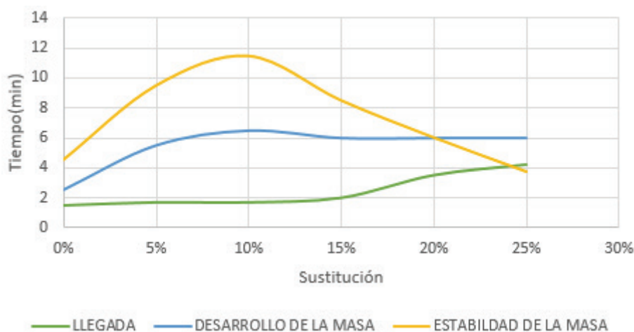
Figura 2: Farinograma
