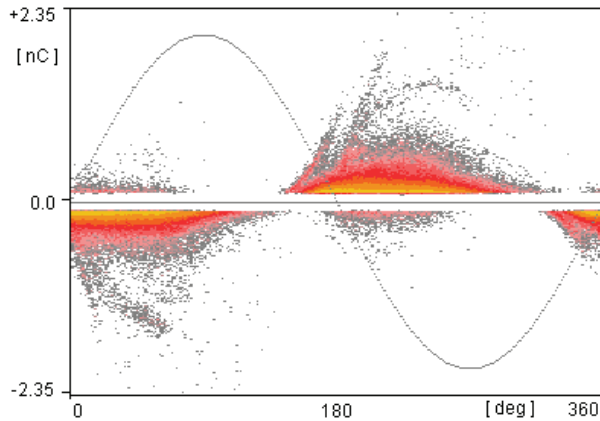
Figura 4. Descarga del tipo interna
