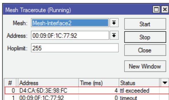
Fig. 6: Mesh traceroute hacia FortiGate 60D
