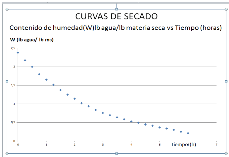
Figura 7: Curva de secado
