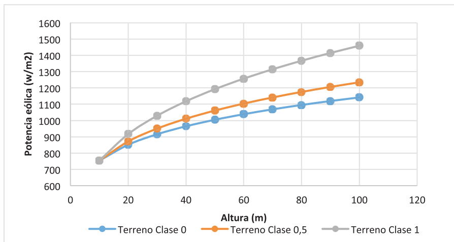
Figura 3. Variación de la potencia eólica disponible (Wattios/m 2 ) con la altura y tipo de terreno
