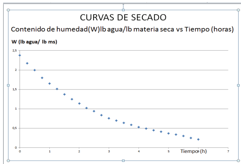
Figura 7: Curva de secado
