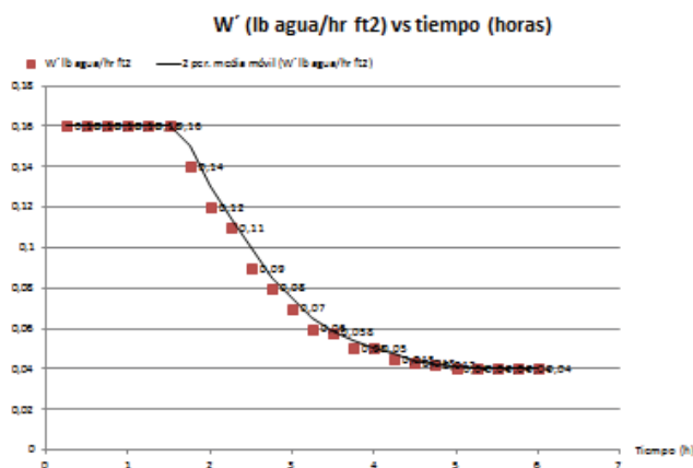
Figura 8: Velocidad de secado vs tiempo de secado
