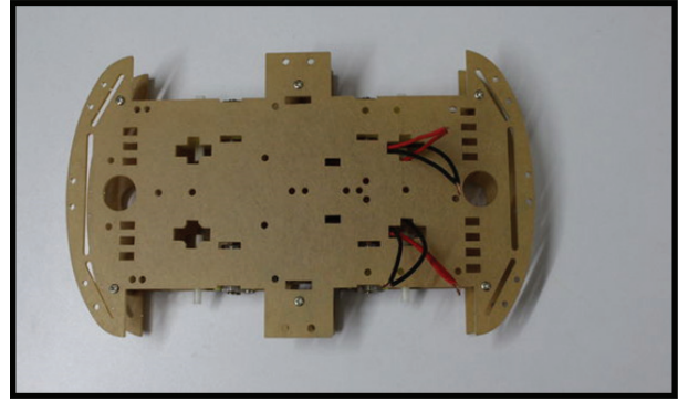
Fig.4: Salida de los cables de los servomotores para su conexión
