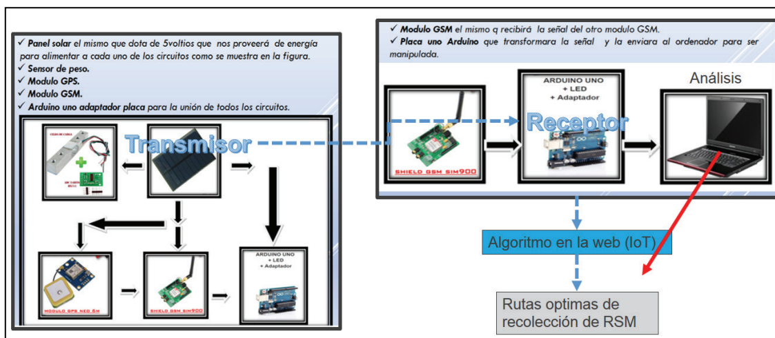
Figura 9. Prototipo para optimizar las rutas de recolección de residuos sólidos urbanos utilizando dispositivos de rastreo satelital e IoT, elaboración propia
