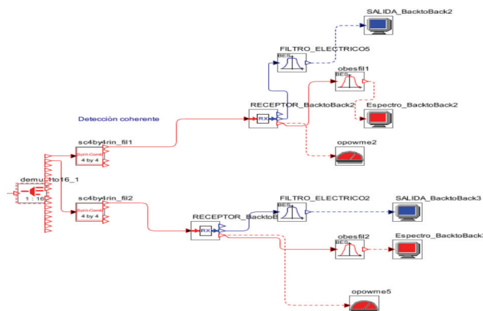
Figura 4. Esquema de detección coherente en el receptor
