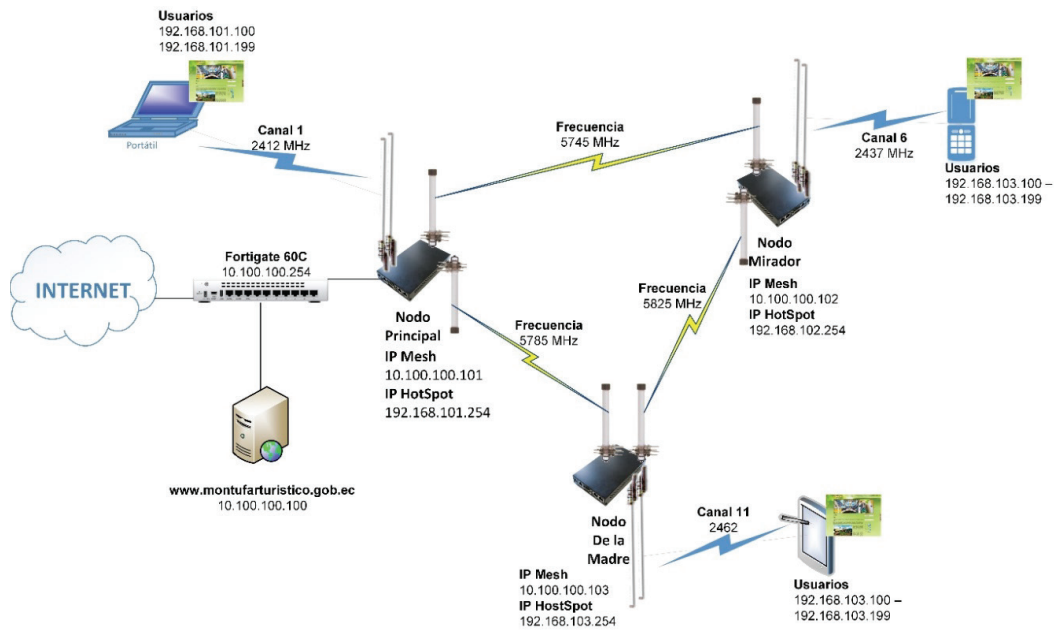
Fig. 2: Diagrama del prototipo
