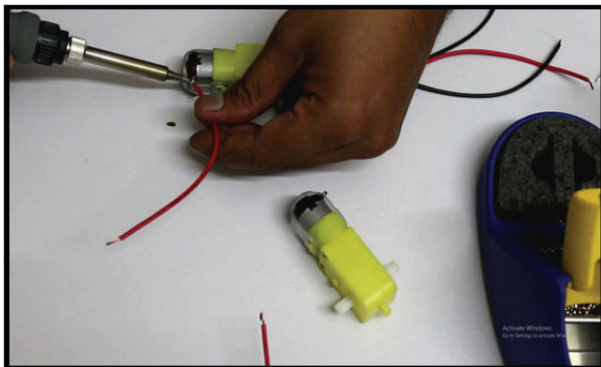
Fig.2: Soldamos los cables a los servomotores
