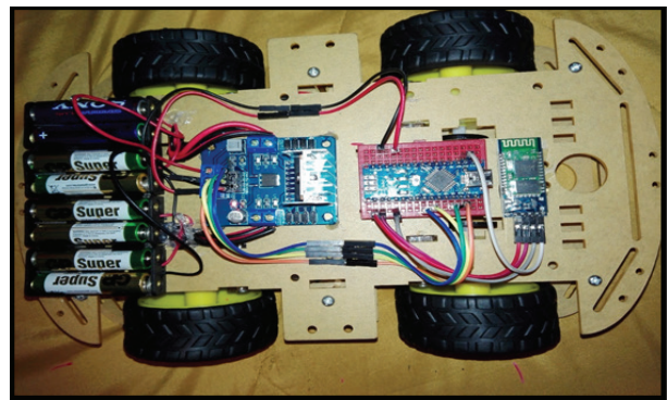
Fig.6: Ensamblaje final der prototipo
