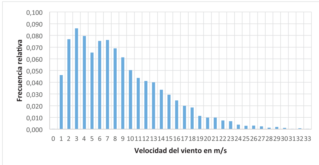
Figura 1. istograma de frecuencias relativas de velocidad del viento
