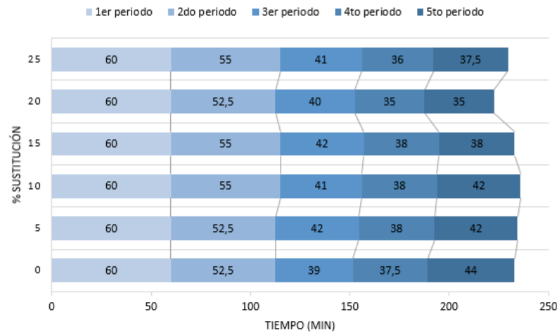
Figura 3. Fermentograma para mezclas de harina de vicia y trigo
