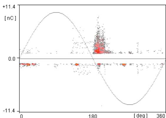
Figura 1. Descarga de tipo ranura
