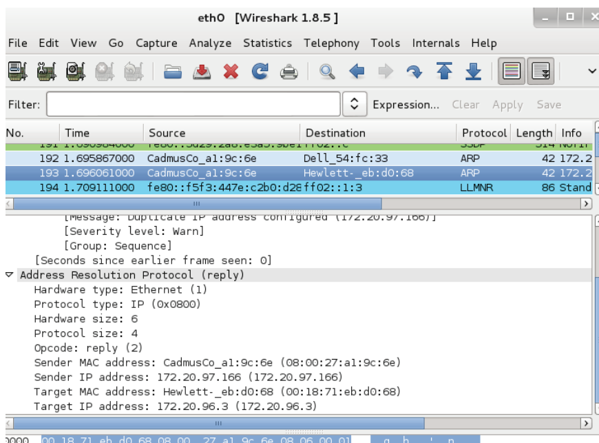
Figura 8: Verificación del protocolo ARP en Wireshark que muestra el ataque ARP Spoffing.
