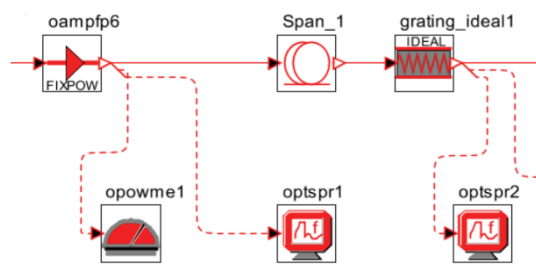
Figura 3. Diseño de un span en el enlace
