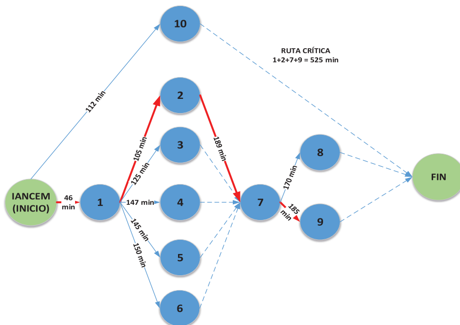
Figura 11. Red de distribución representada como un grafo
