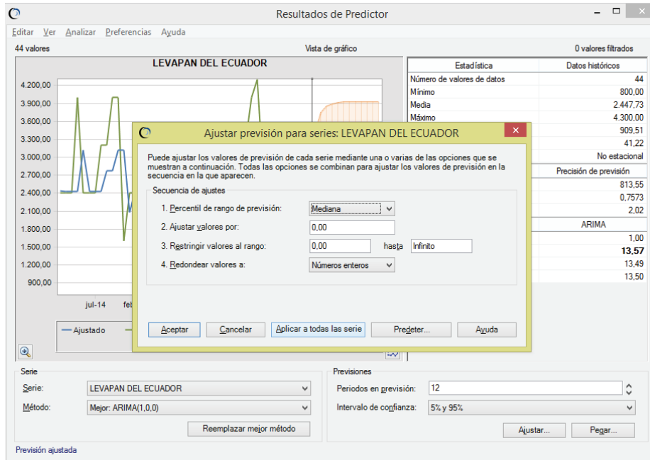
Figura 9. Ajustes en los pronósticos
