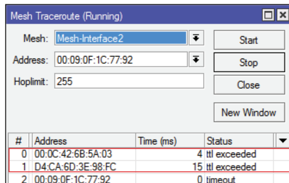
Fig. 10: Mesh traceroute hacia FortiGate 60D con cambio de topología
